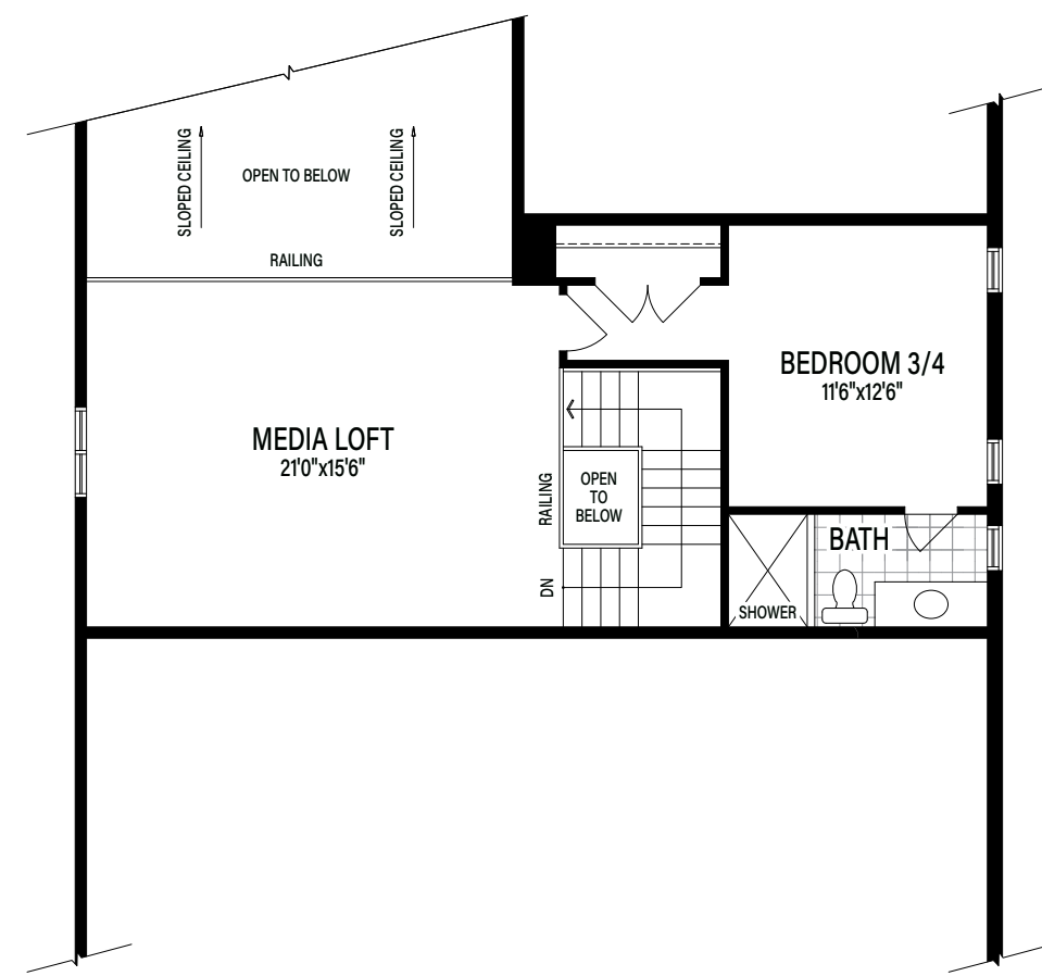
Optional Loft Elevation A (B & C Similar)
