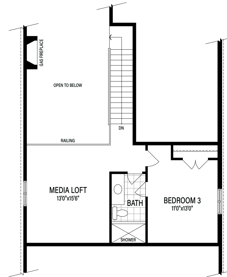
Optional Loft Elevation A (B & C Similar)
